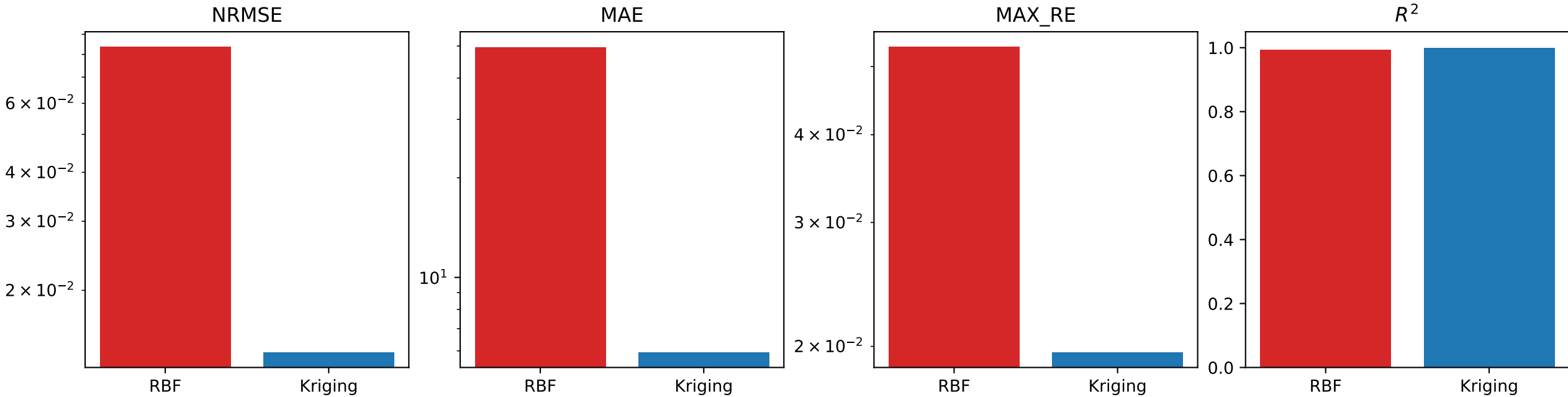
Якість RBF vs Kriging при n_s = 50 на RD-2D / J
